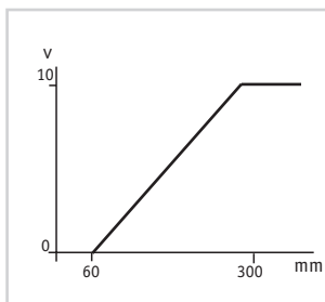
Uscita analogica in tensione Power voltage analogical output
