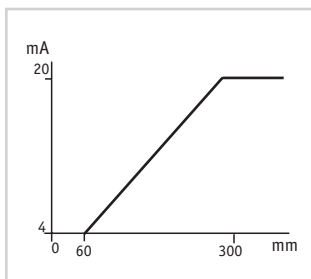
Uscita analogica in corrente Current analogical output
