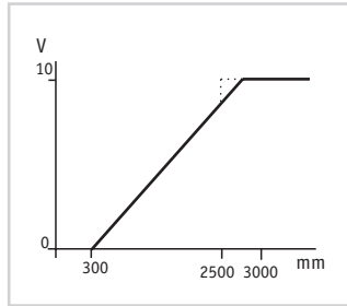
Uscita analogica in tensione Power voltage analogical output
